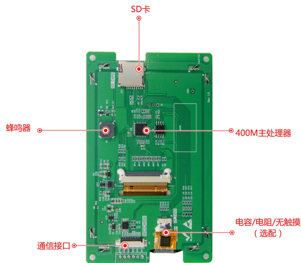
图 1-4 硬件配置图
