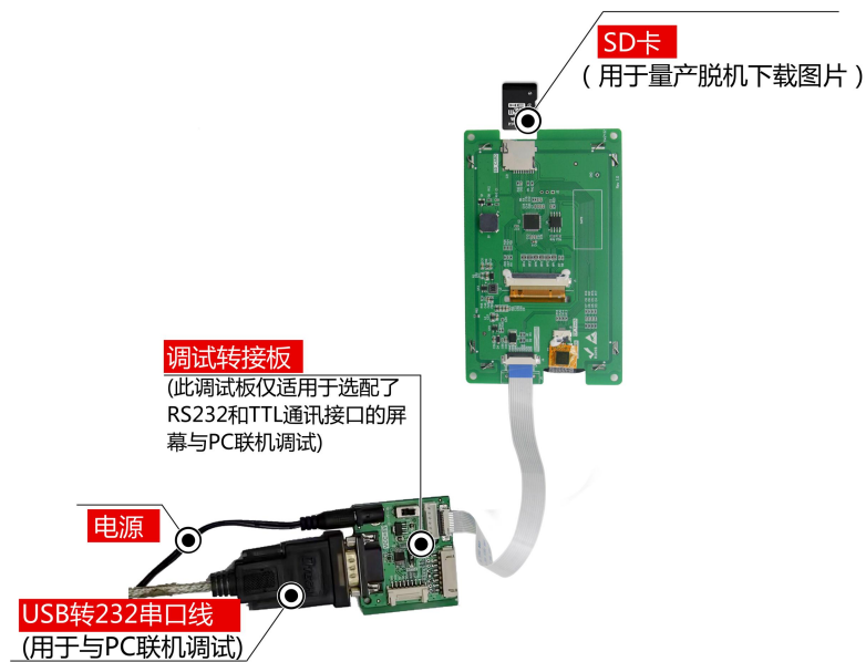
图 1-5 调试工具图
